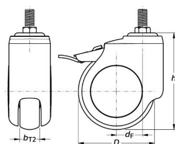
Kastor Hidup TPRJB dengan Rem Total
