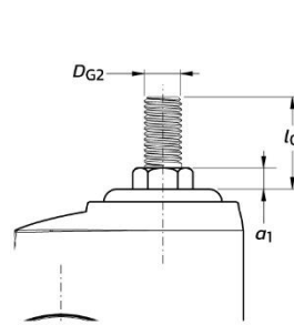
Kastor dengan Single Bolt Fixing (akhiran BF58)
