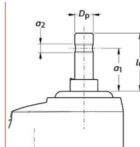
Kastor dengan Solid Stem Fitting (akhiran SF16)
