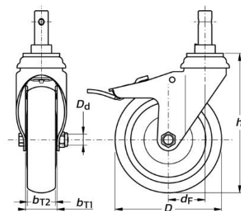
Kastor Hidup TPRJB dengan Rem Total
