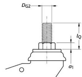
Kastor dengan Single Bolt Fixing (akhiran BF58)
