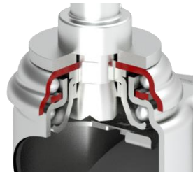
Bantalan penahan beban yang terbuat dari hardened steel (divisualisasikan dengan warna merah)
