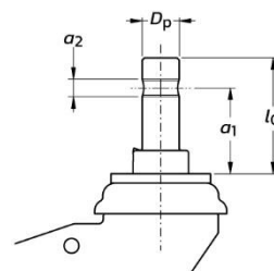
Kastor dengan Solid Stem Fitting System (akhiran SF16)
