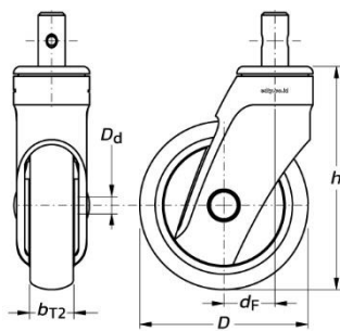
Kastor Hidup TPRJ
