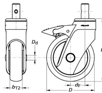
Kastor Hidup TPRJB dengan Rem Total
