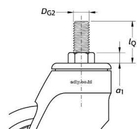
Gambar berlaku untuk kastor dengan pengepasan baut tunggal (akhir BF58, BF12, atau BFM12)
