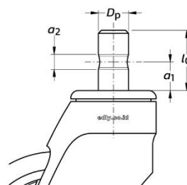
Gambar berlaku untuk kastor dengan pengepasan as dengan lubang ulir (akhir SF20 atau SF32)
