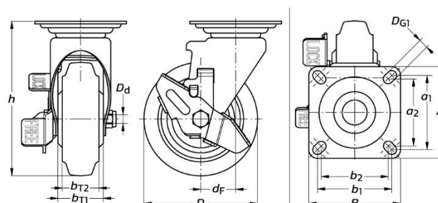
Kastor Hidup NBK (berlaku untuk rangka kastor dengan atau tanpa rem roda)
